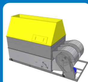
Выпускной колпак
