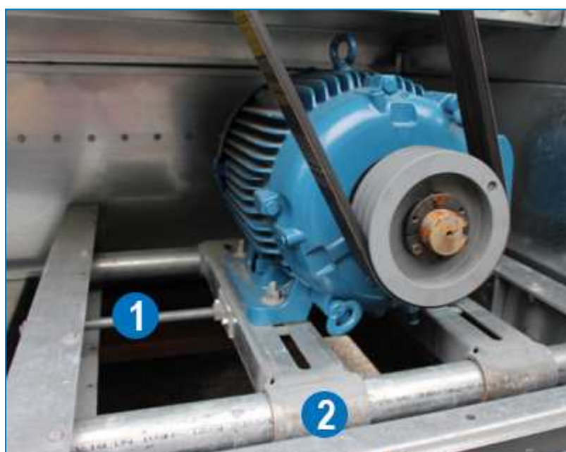
Verstelbare motorbasis
