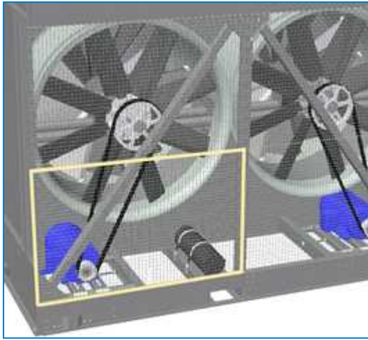
Onderste ventilatorafscherming
