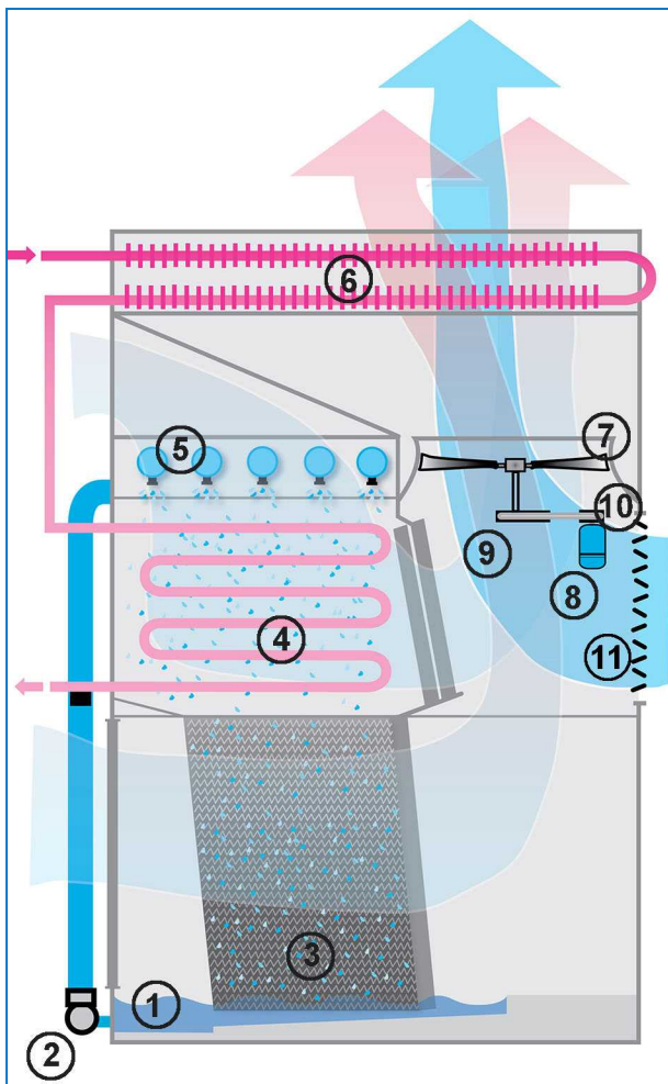
Werkingsprincipe - Open modulerende luchtinlaatdempers
